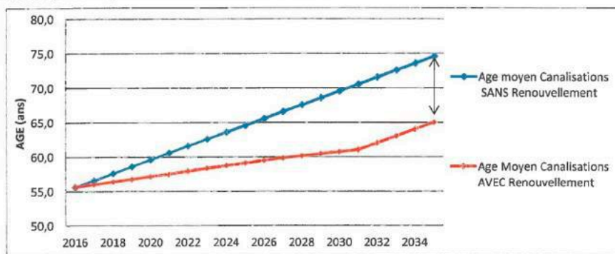
Titre : Evolution de l'âge moyen du réseau avec et sans renouvellement (Taux moyen de renouvellement = 1%/an pendant 15 ans)
