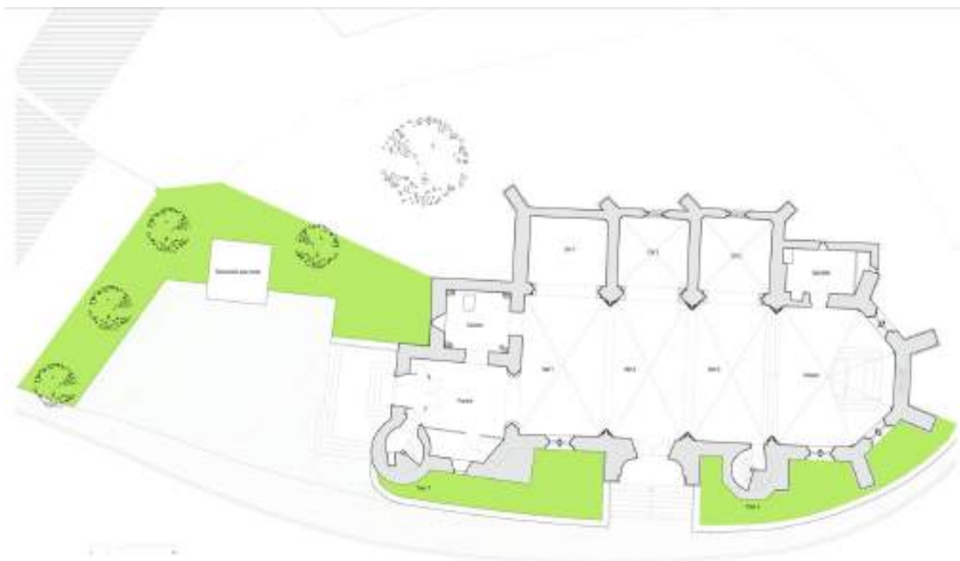
Plan général projeté de l'église Saint Laurent
